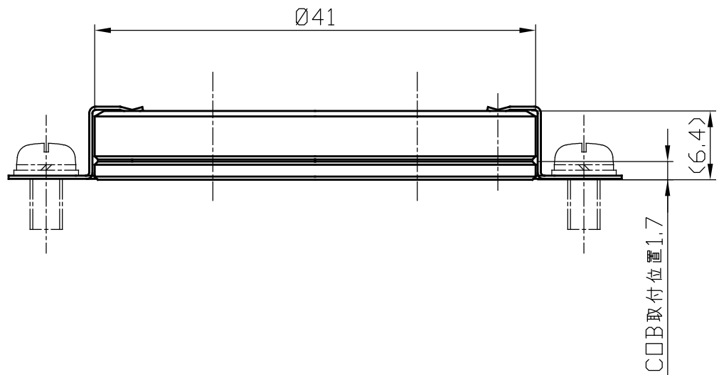
品名 : COB-C1919SC ソケット
